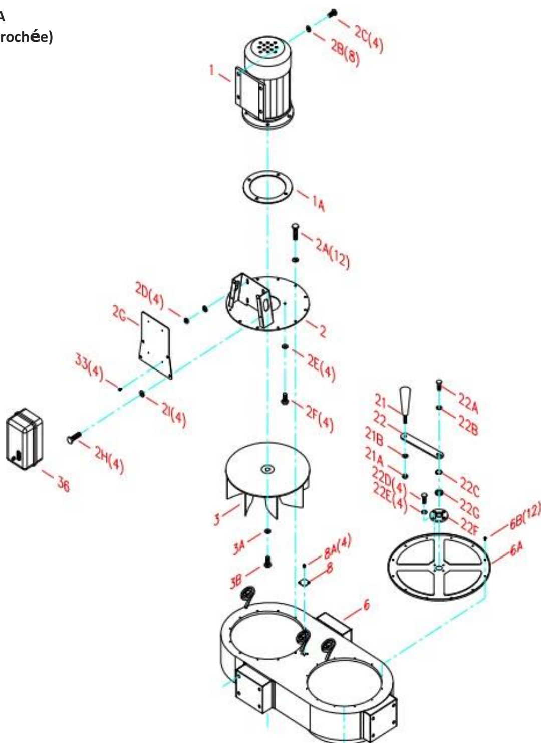
Figure 48 : Ventilateur, moteur et interrupteur
