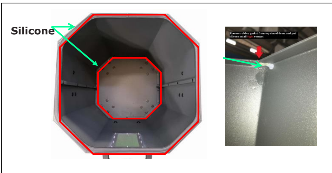
Figure 29 : Sceller le tambour avec du silicone (impératif!)
