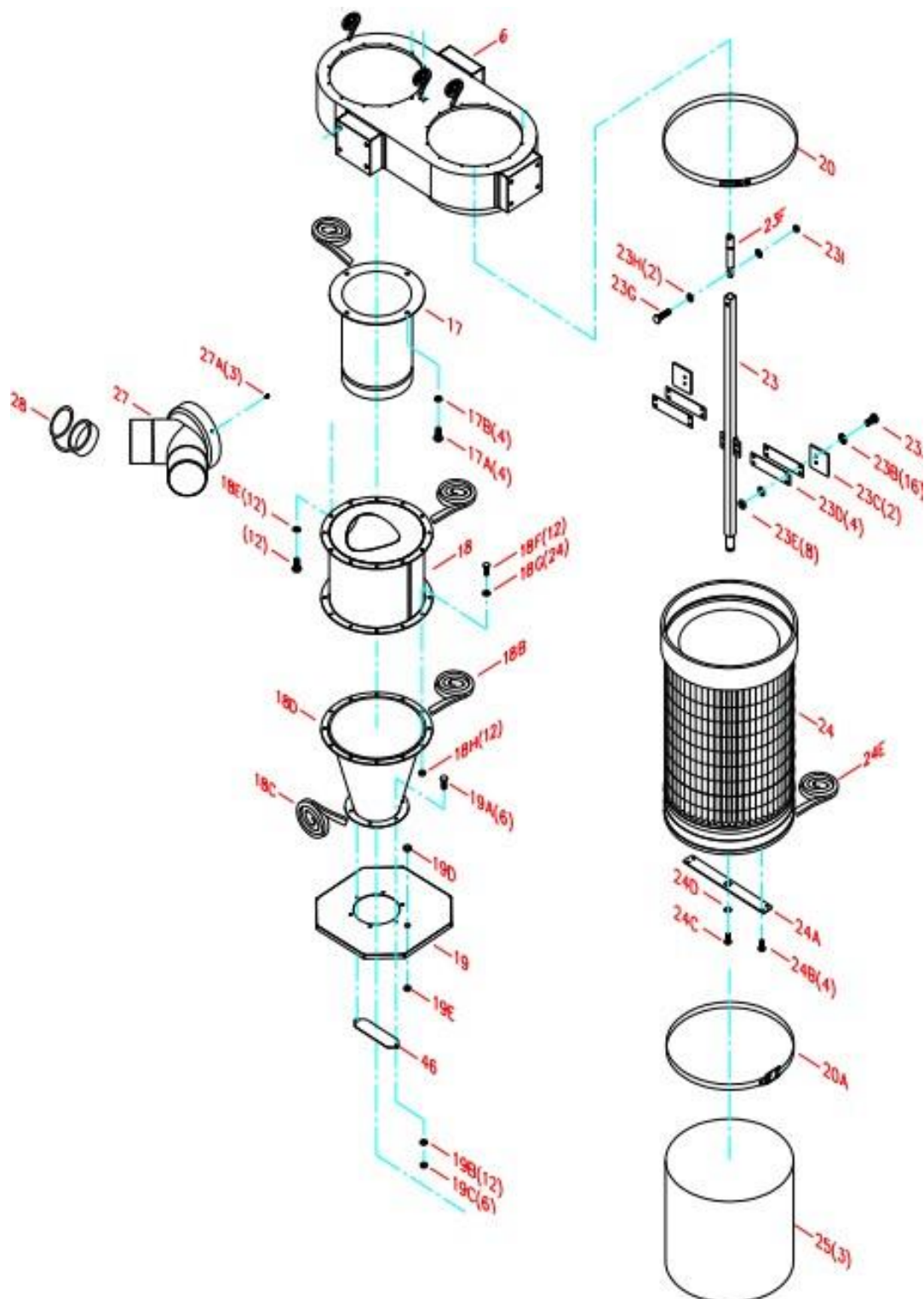
Figure 49 : Cyclone, filtre extérieur et tonneau
