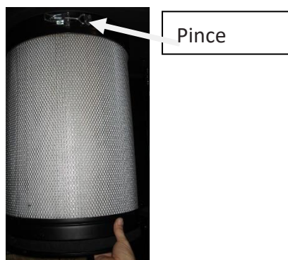
Figure 44 : Tenir le filtre extérieur par le bas lors du desserrage de la pince (en haut)
