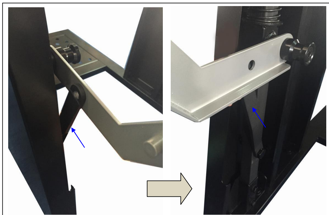
Figure 21 : Alignement du support et de la pédale de commande
