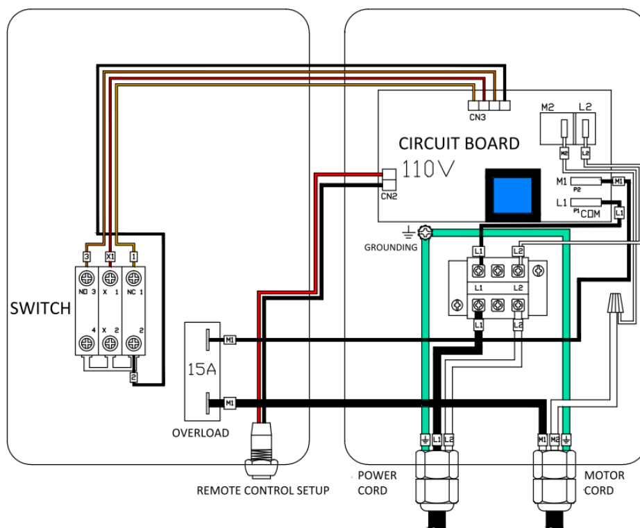
Figure 2 : Câblage interne
