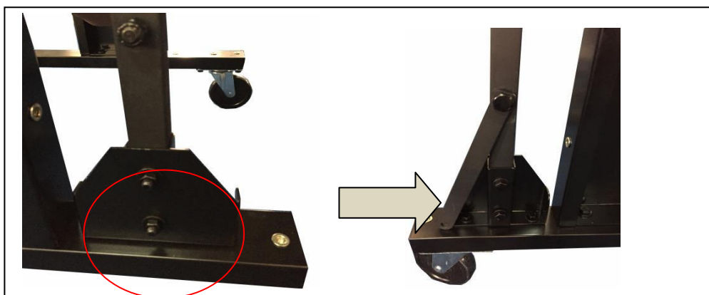
Figure 17 : Fixation de la base de la barre de pédale
