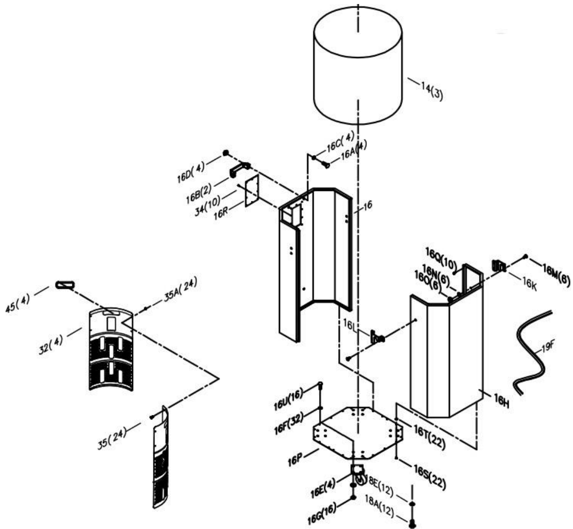
Figure 51 : Canon et insert
