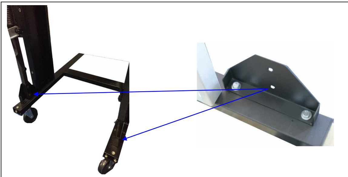
Figure 14 : Fixation de la plaque triangulaire inférieure
