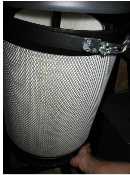
Figures 45-46 : Démontage du filtre extérieur pour le nettoyage
