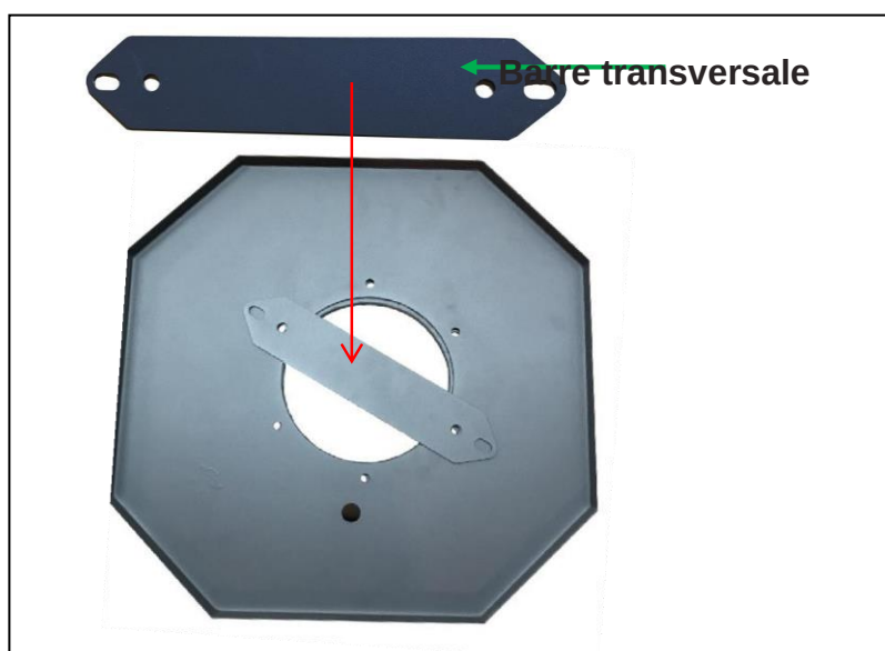
Figure 23 : Fixation de la barre transversale au couvercle du tambour
