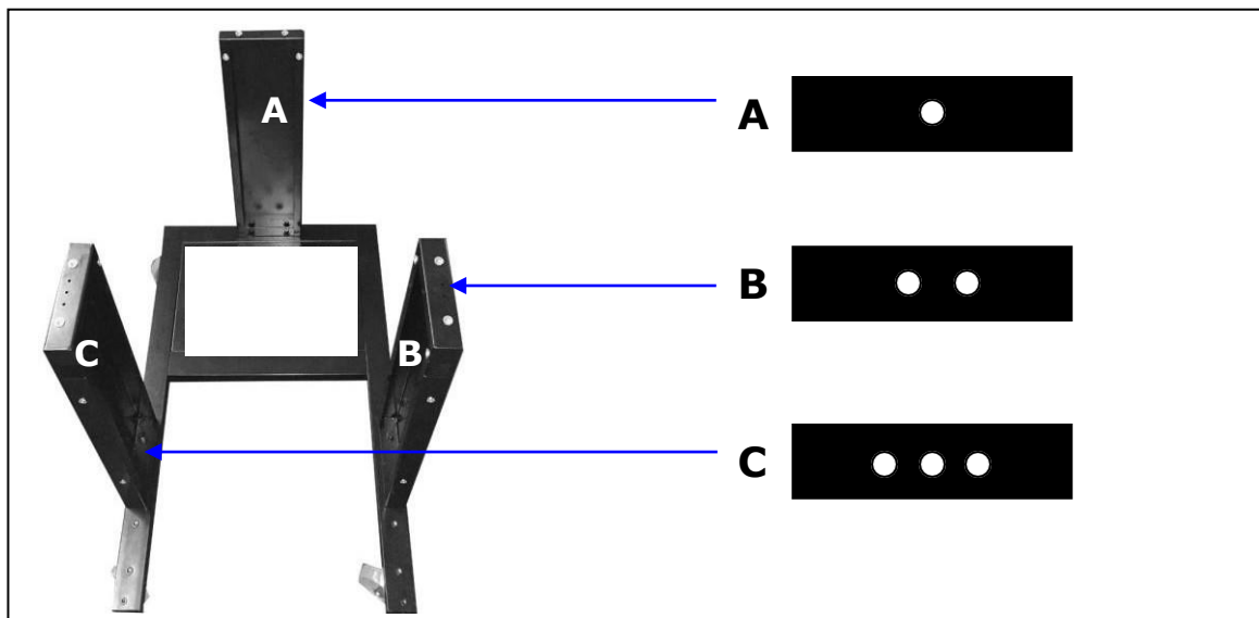
Figure 10 : Fixation des panneaux de support à la base
