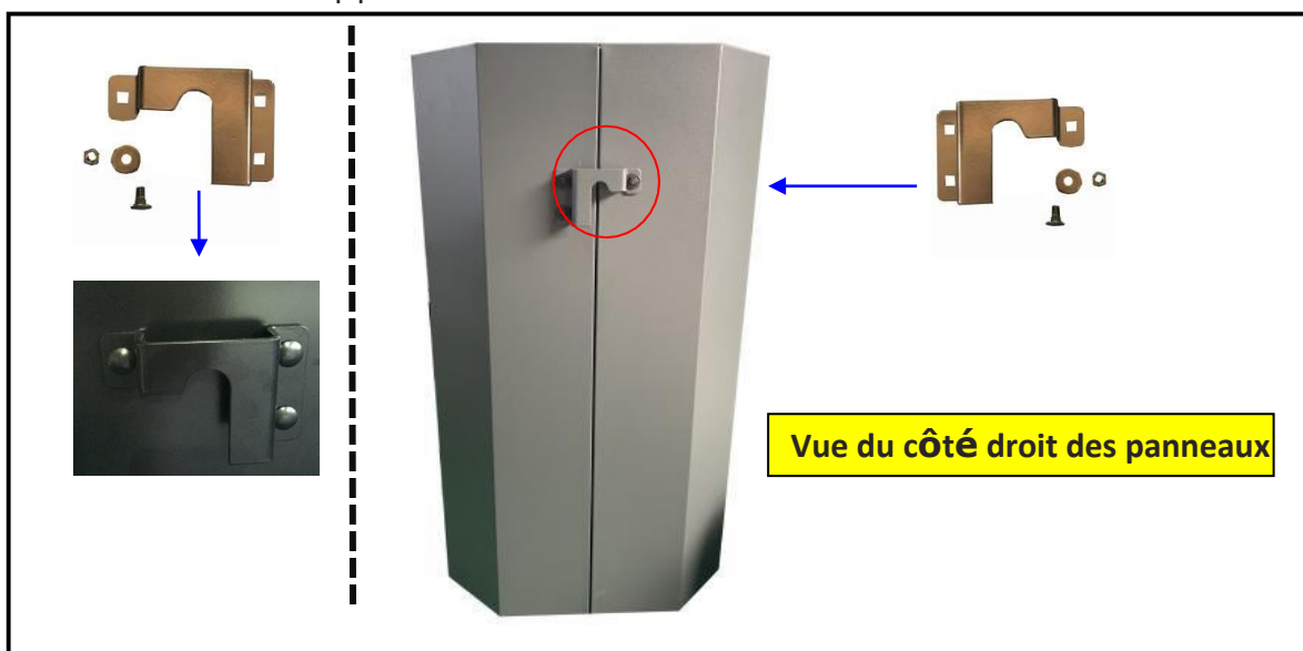
Figure 27 : Fixation des plaques latérales au tambour
