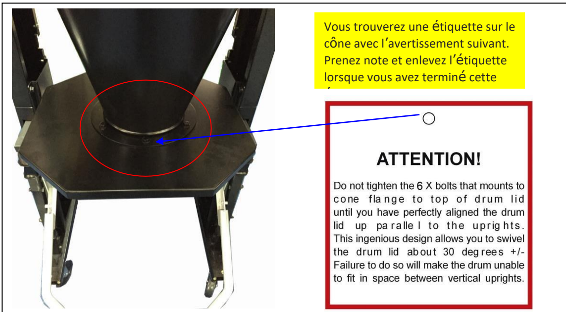
Figure 24 : Application de la bande de mousse et fixation du couvercle du tambour
