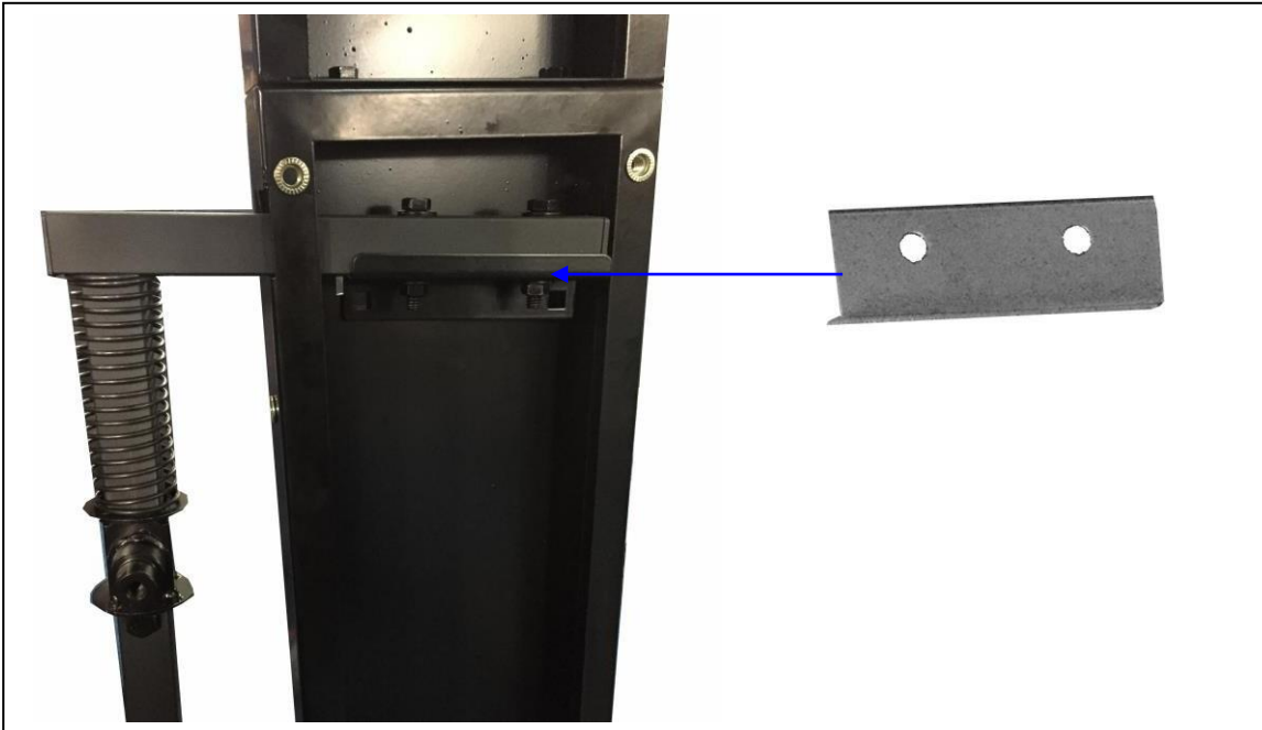
Figure 16 : Fixation du support de la pédale
