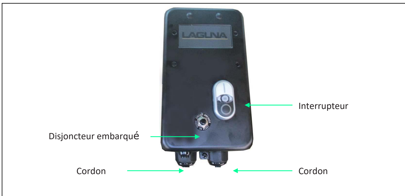
Figure 39 : Interrupteur manuel avec récepteur de télécommande à haute fréquence
