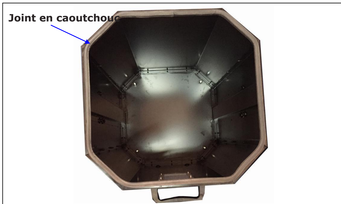
Figure 31 : Fixation du joint au tambour octogonal
