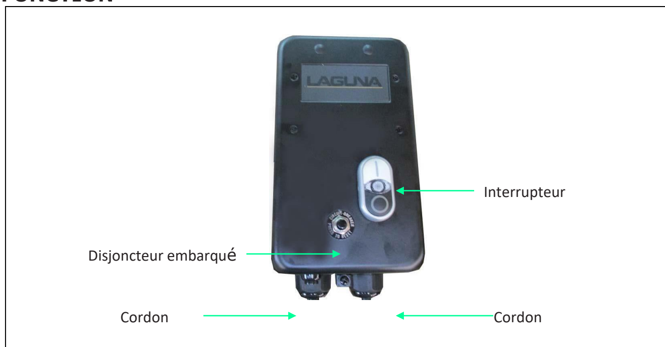
Figure 3 : Récepteur de télécommande à haute fréquence et interrupteur manuel
