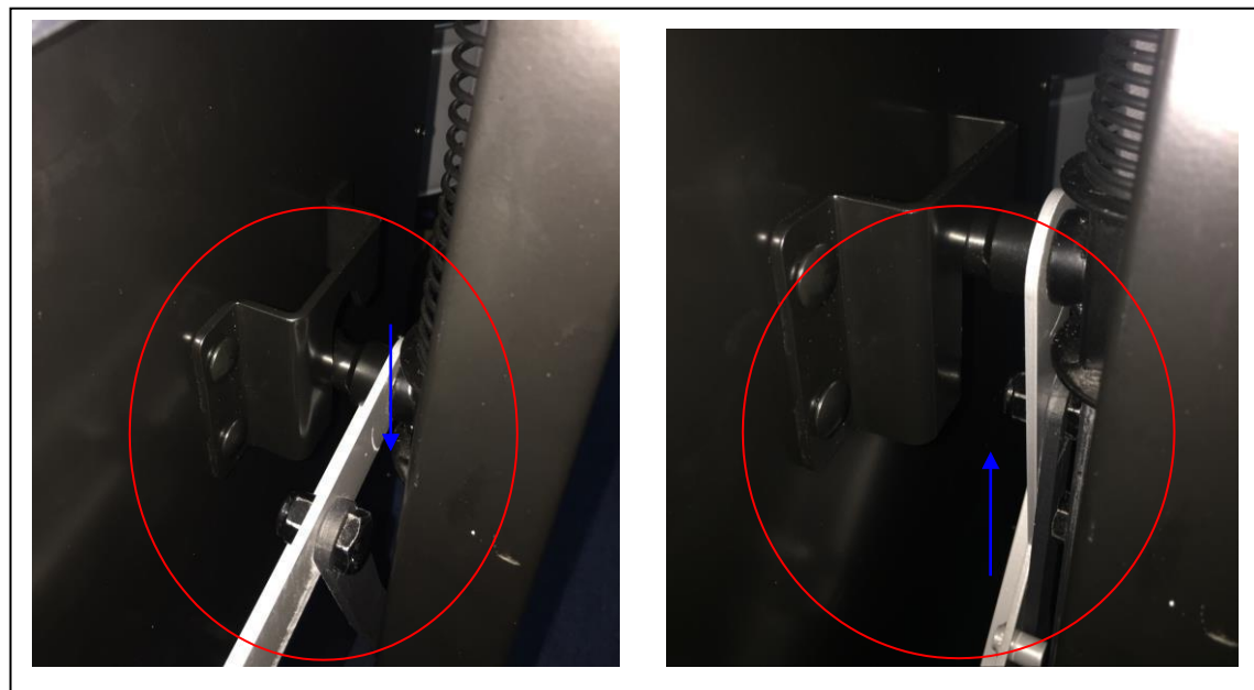
Figure 35 : Confirmation de l'emplacement de la plaque de levage
